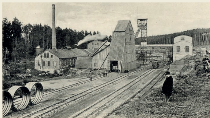
Ansicht der Schachtanlage, Westseite, März 1900 Schacht Marie und Schacht Julius.
